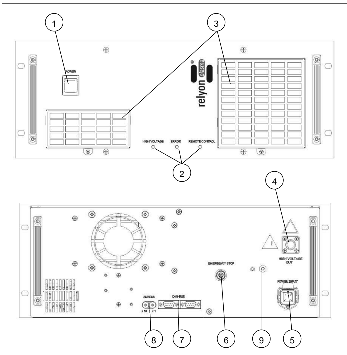
Fig. : Représentation schématique de la face avant (haut) et de la face arrière (bas) du bloc d'alimentation PS2000
