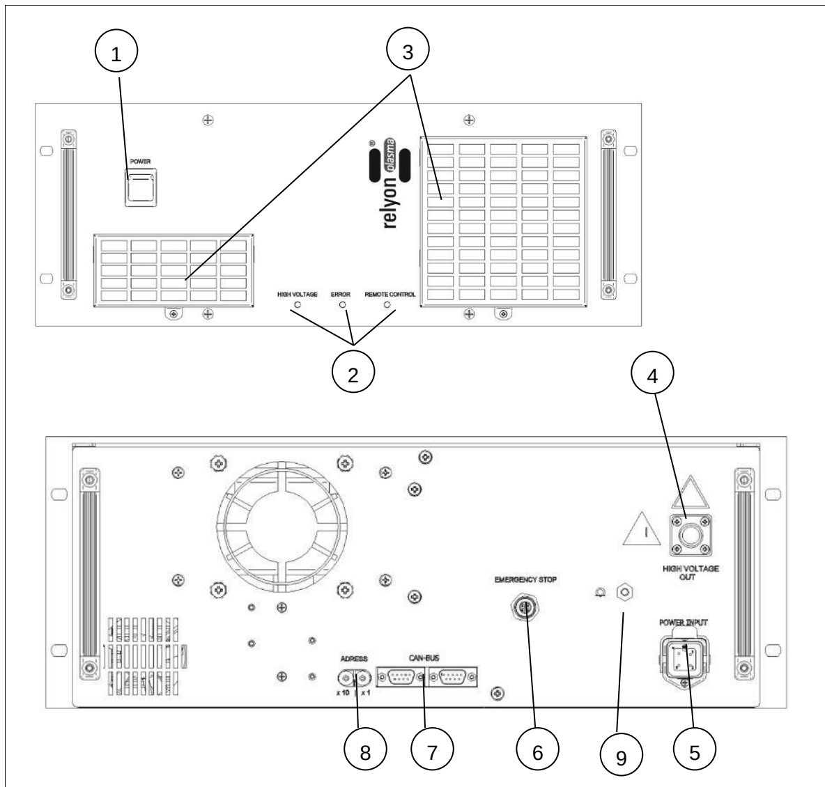
Fig.: Representación esquemática del lado delantero (arriba) y trasero (abajo) del PS2000
