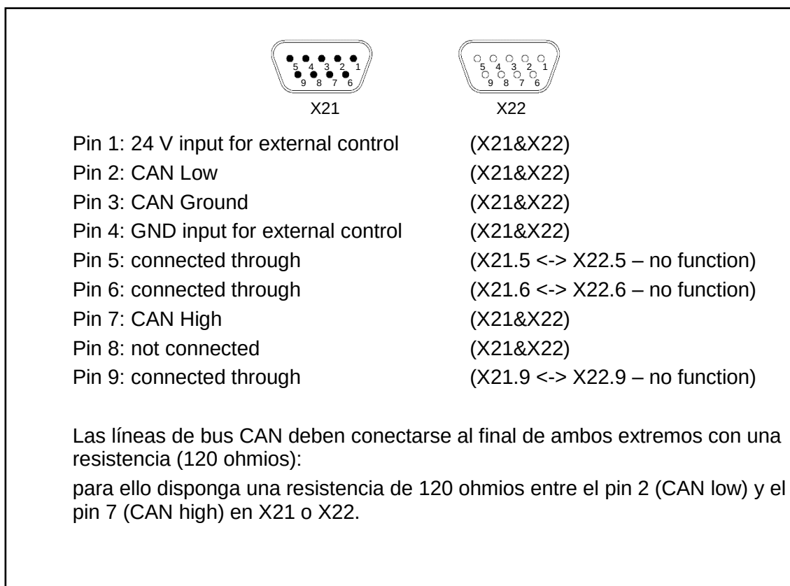
Fig.: Asignación de conexiones de la hebrilla/el conector Sub D (izquierda) así como representación esquemática de las dos interfaces (derecha).
